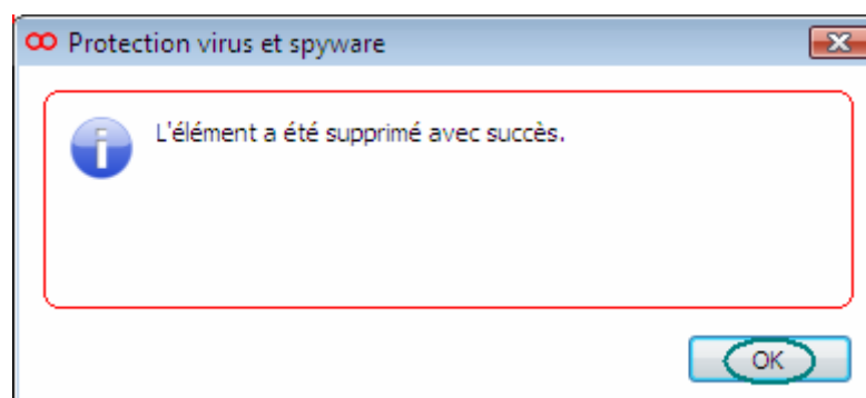
Figure 4 : Rootkit supprimé
